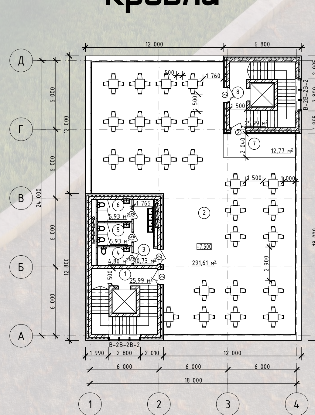
План эксплуатируемой кровли
