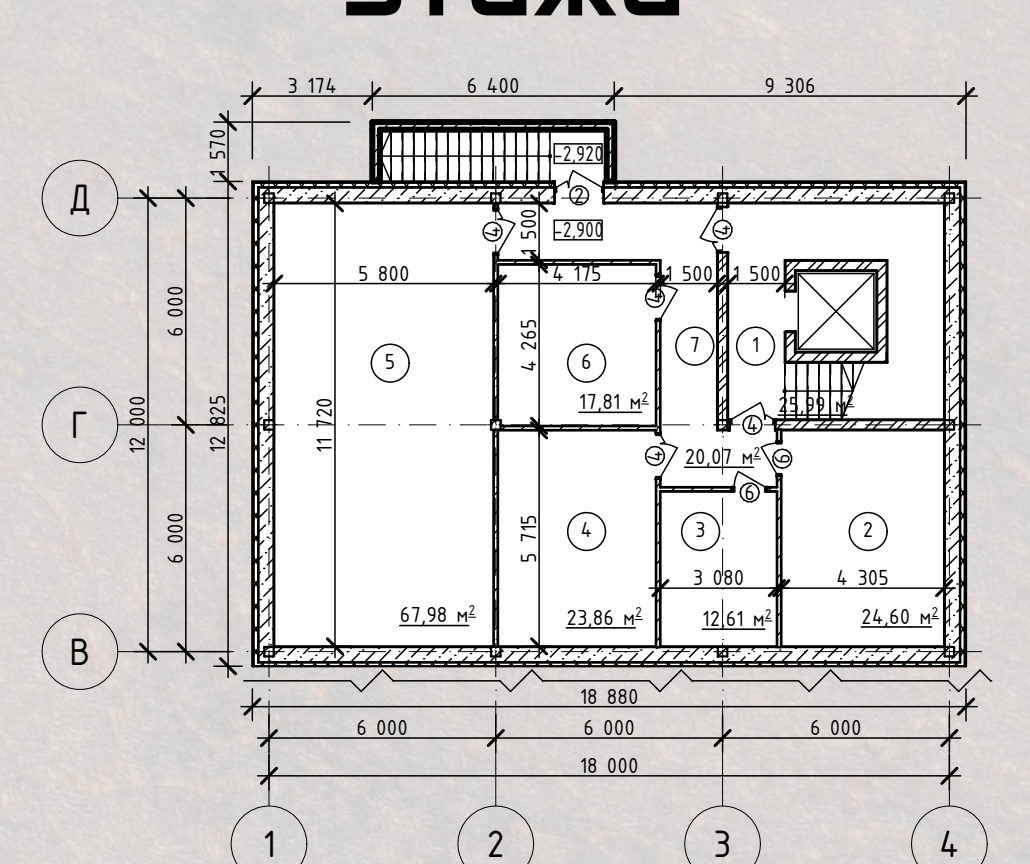
План подвального этажа
