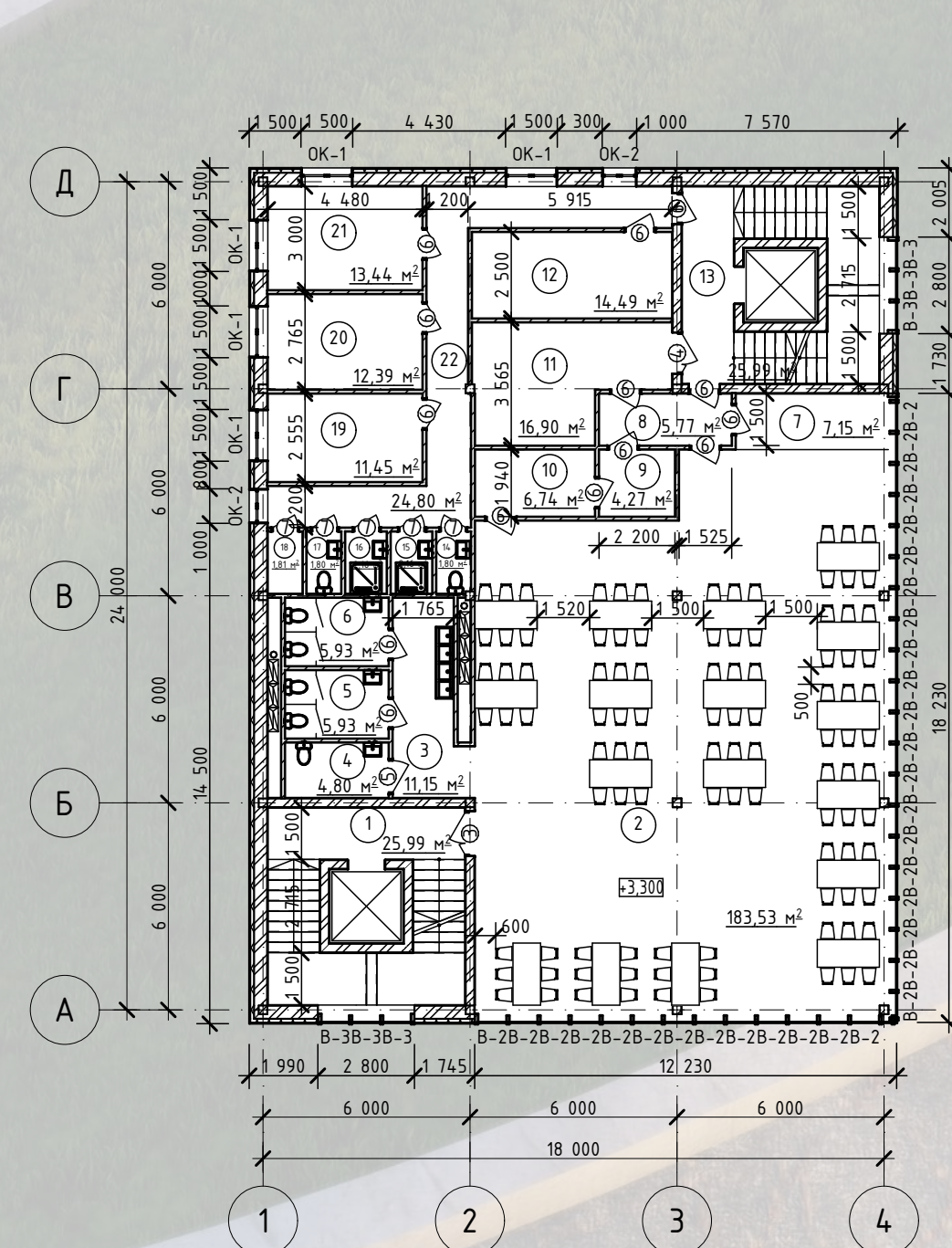
План 2-го этажа
